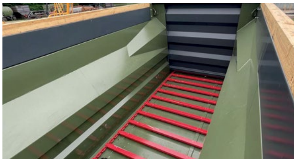
Przeñośnik łańcuchowy o szerokości 1,3 m
